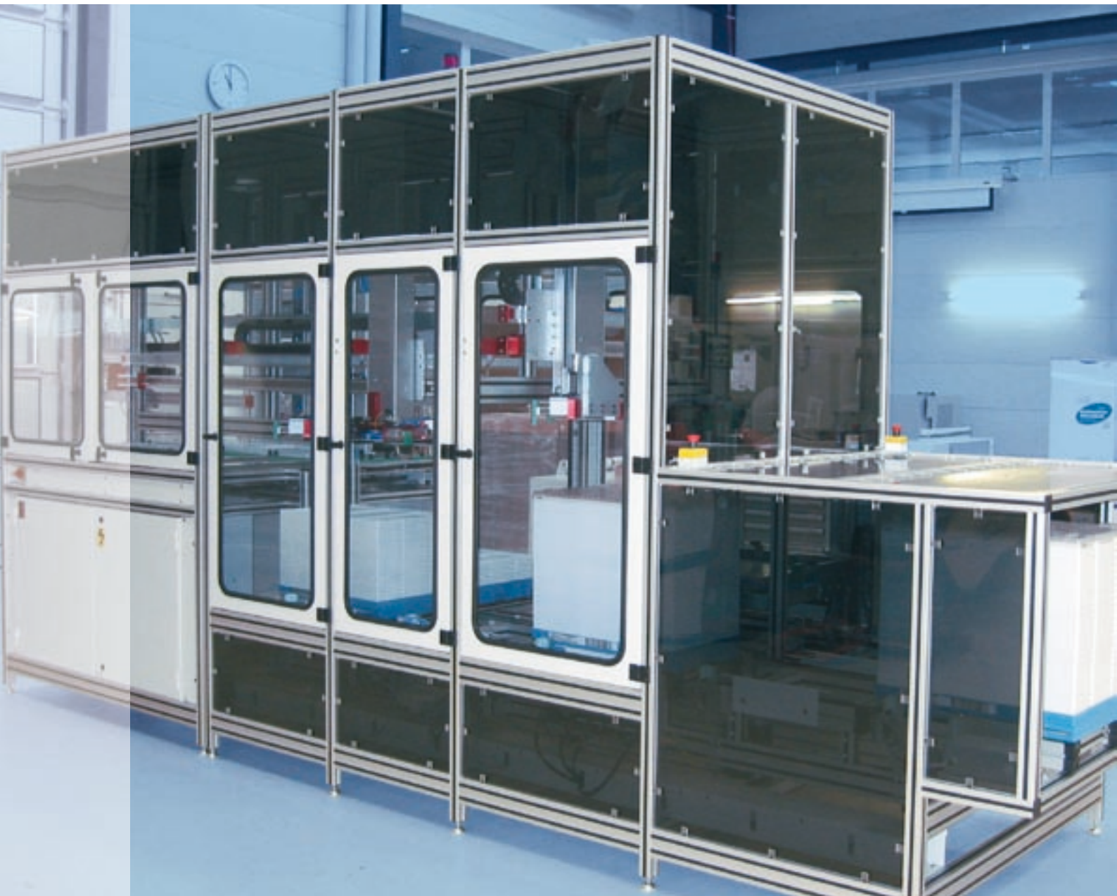
Cabina di montaggio flessibile per la produzione di orologi Célula de montaje flexible para la producción de relojes Célula de montagem flexível para a produção de relógios Humard Automation SA, Delemont, CH
