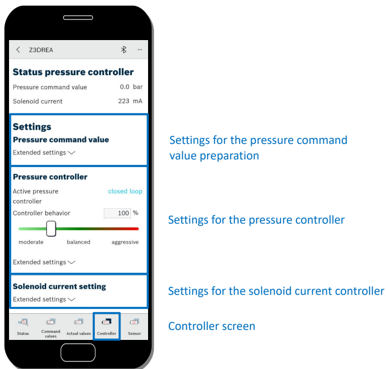
Fig. 46: Controller structure4
