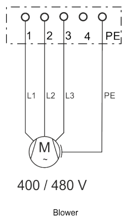
Fig. 366: MS2N Fan connection 400 / 480 V
