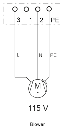
Fig. 364: MS2N Fan connection 115 V
