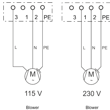
Fig. 386: MS2N Fan connection 115/ 230 V
