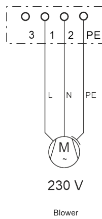
Fig. 365: MS2N Fan connection 230 V
